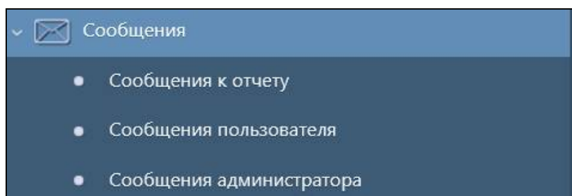
Рисунок 1 – РМ «Сообщения»
